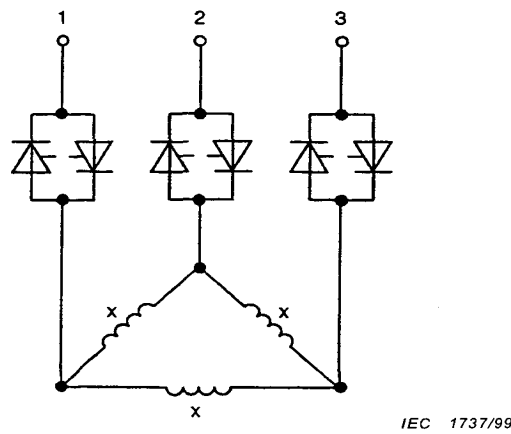
Figure 2c – Moteur en triangle – Thyristors raccordés entre le bobinage et l'alimentation
