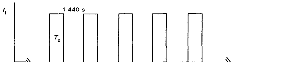
Profil du courant d'essai pour AC-52b, AC-53b, AC-58b
