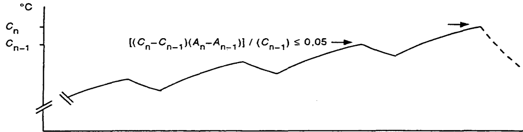
Profil standard d'élévation de température
