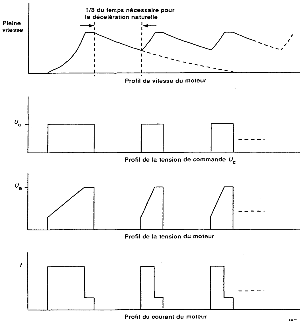
Figure F.3 – Profil d'essai de capacité de blocage et d'aptitude à la commutation
