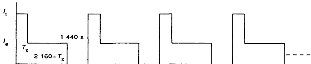
Profil du courant d'essai pour AC-52a, AC-53a, AC-58a
