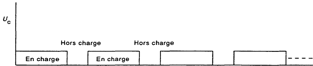
Profil standard de la tension de commande U_c
