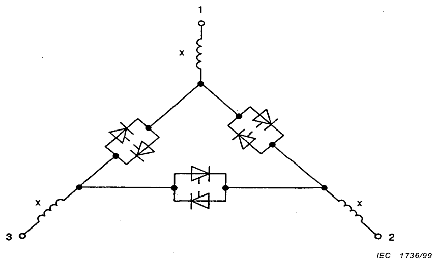
Figure 2b – Moteur en étoile – Thyristors en triangle
