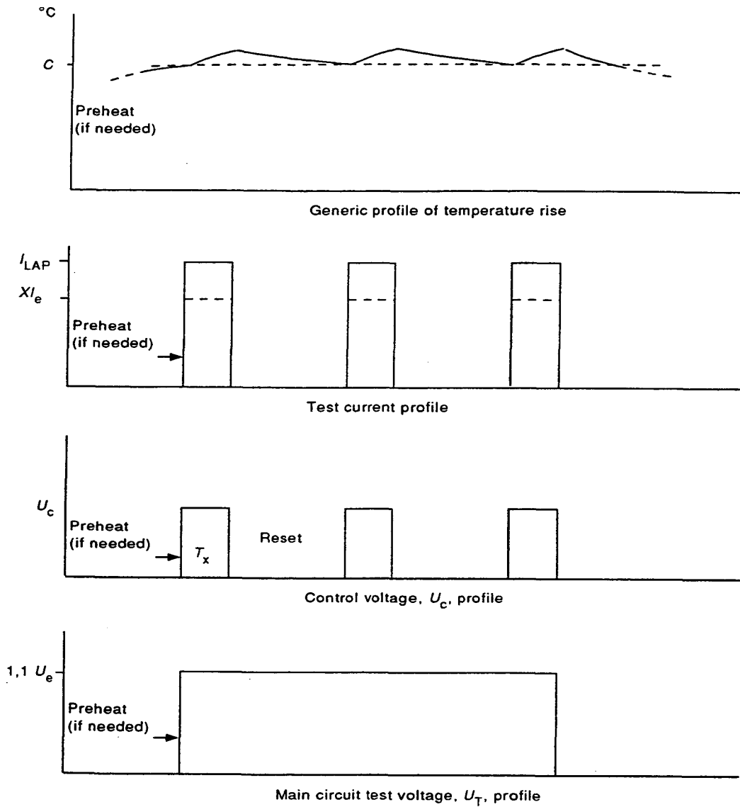
Figure F.2 – Profil d'essai de capacité de surcharge
