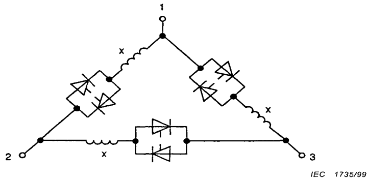
Figure 2a – Moteur en triangle – Thyristors en série avec un bobinage
