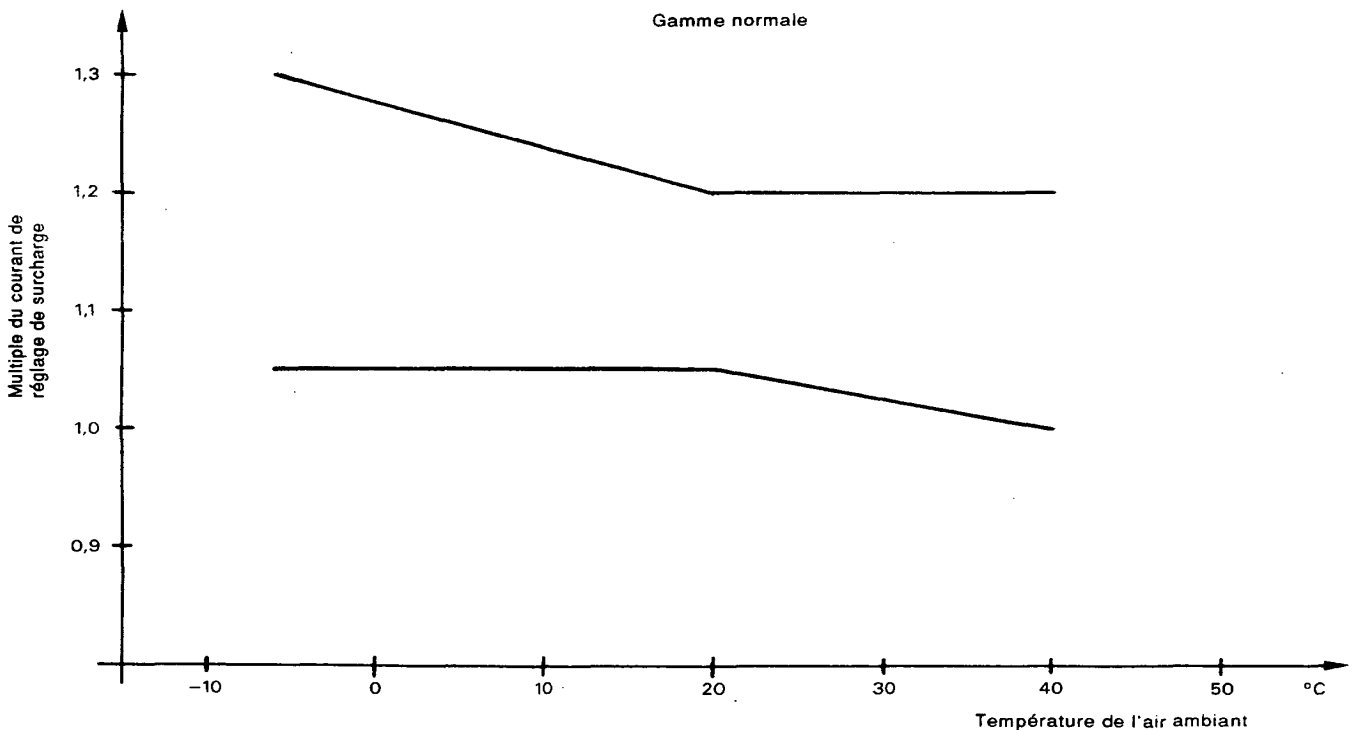
Figure B.1 – Multiple des limites de courant de réglage pour les relais de surcharge temporisés compensés pour les variations de température de l'air ambiant
